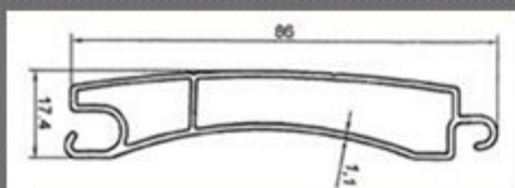
77 mm SLAT: Extruded profile Ekstrüzyon profili Ekstruzni profil
